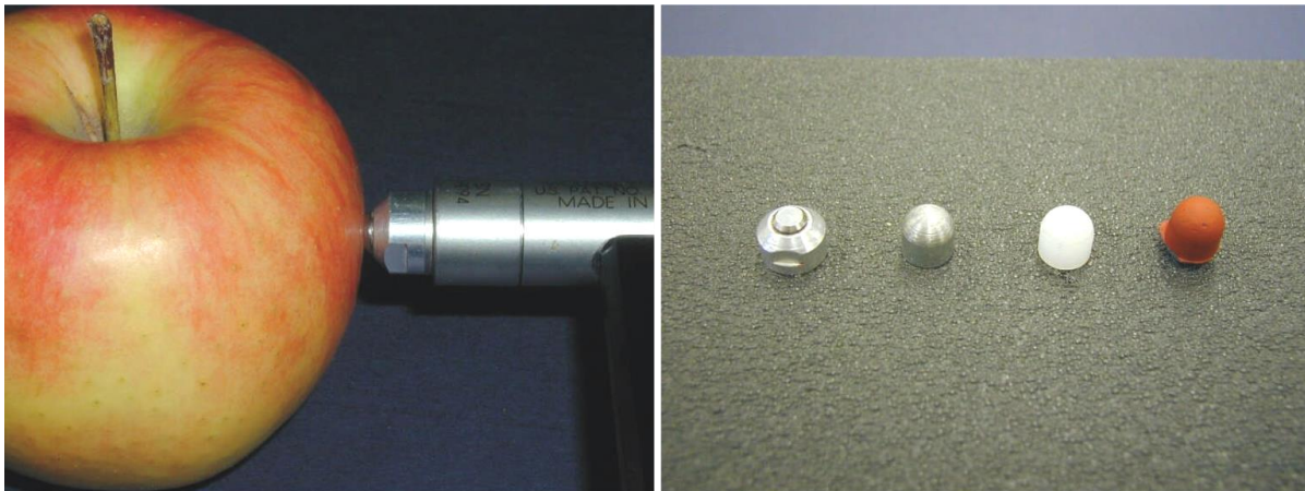
2.19. ábra Vizsgált ütőfej alakok- és anyagok roncsolást nem okozó mechanikai impulzus nagyságának meghatározásához (Felföldi, 2004)
