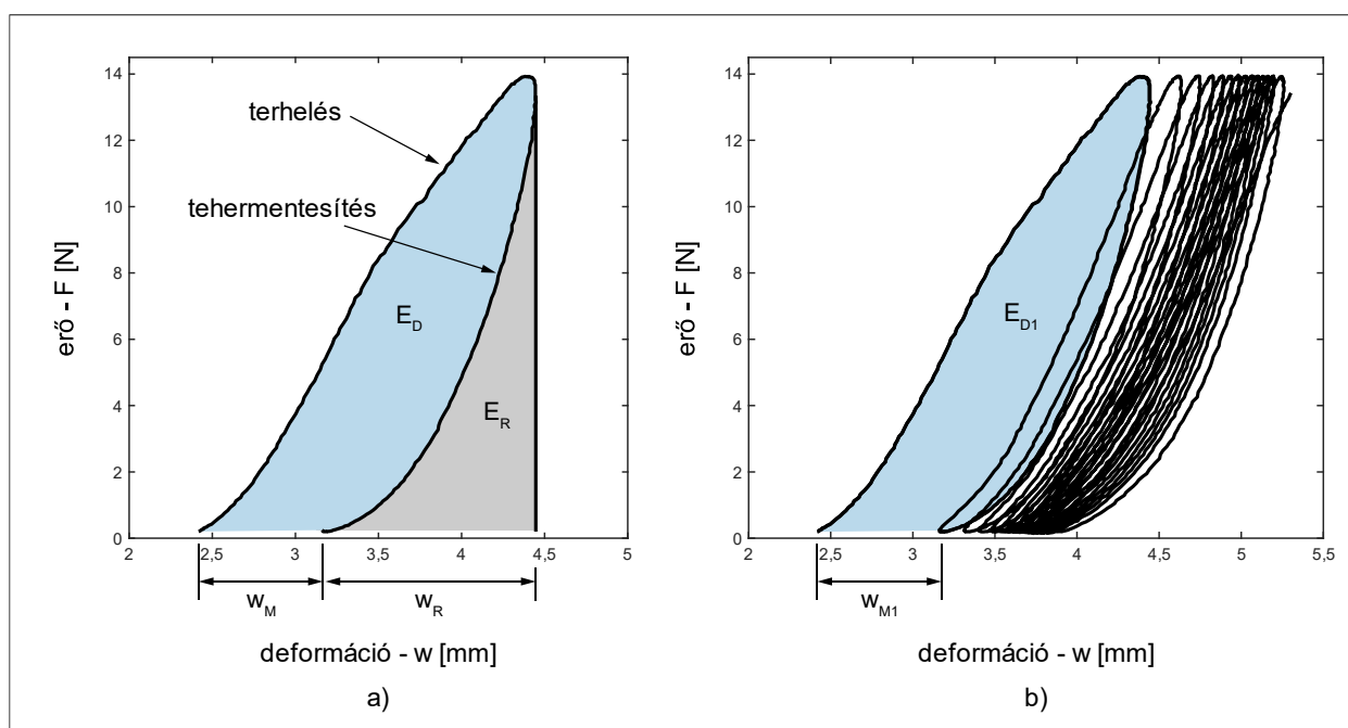
3.21. ábra Egy terhelési ciklus erő-deformáció görbéje, valamint a termény erő-deformáció görbéje a tönkrementelig egy Golden Delicious alma esetén
