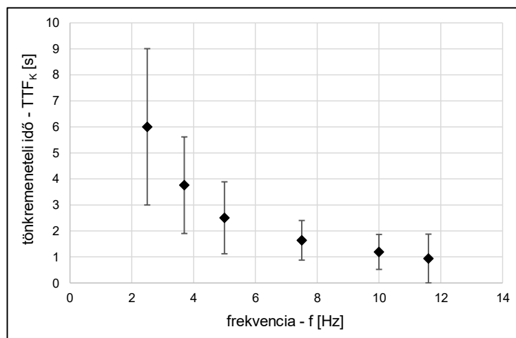
4.1. ábra A külső töréspontig eltelt időtartamok frekvenciafüggése Golden Delicious almák esetén
