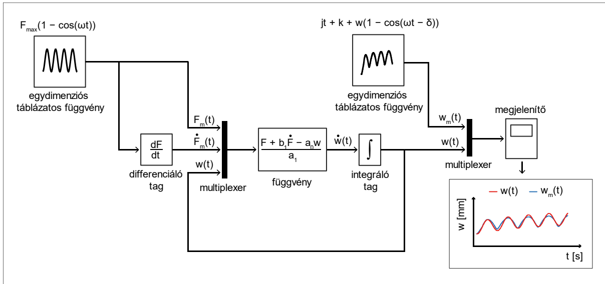
3.18. ábra Simulink szabályozókör működése
