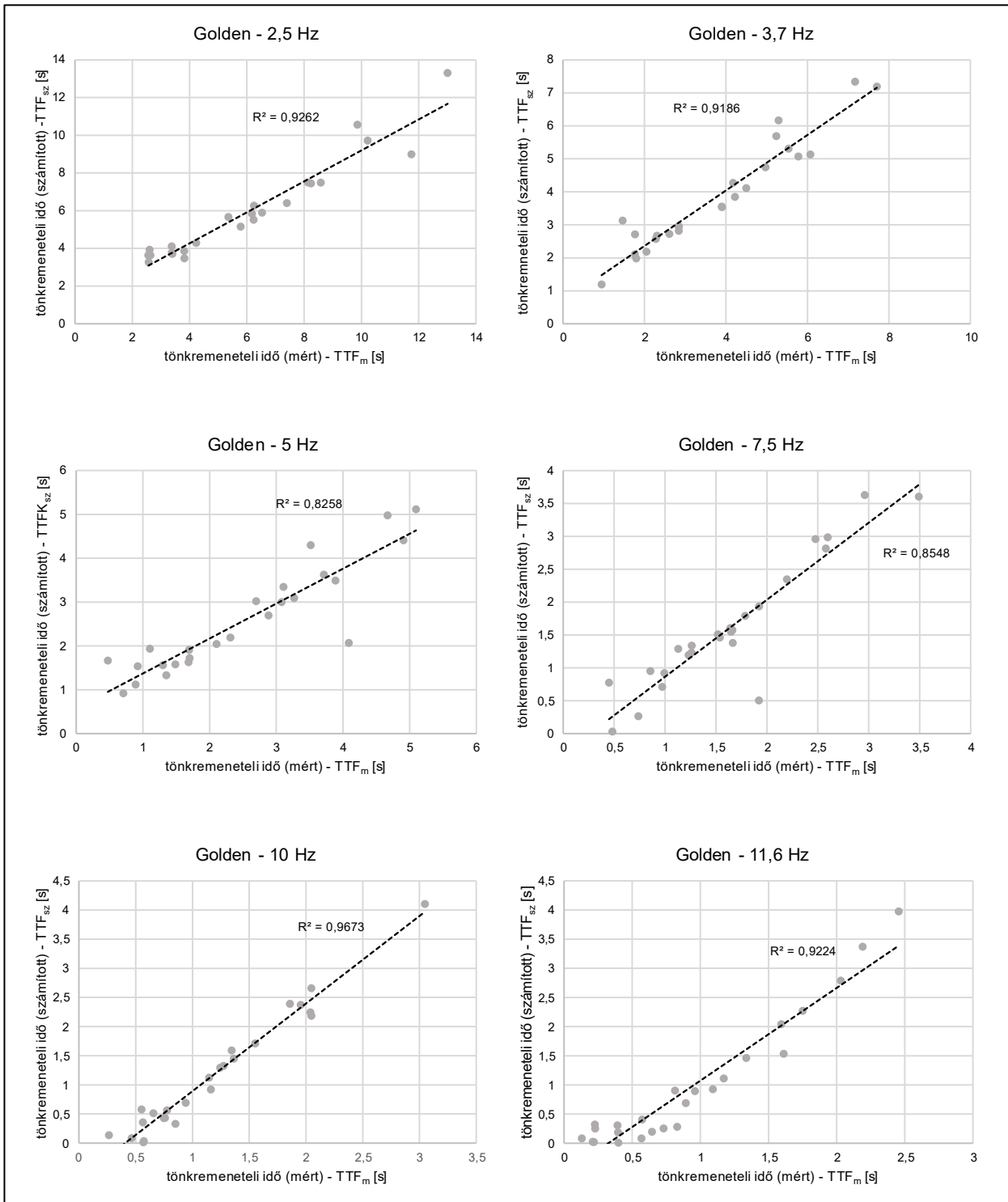
8.1. ábra Mért és számított tönkrementeli időtartamok kapcsolata az egyes frekvenciabeállításokon Golden Delicious almák esetén
