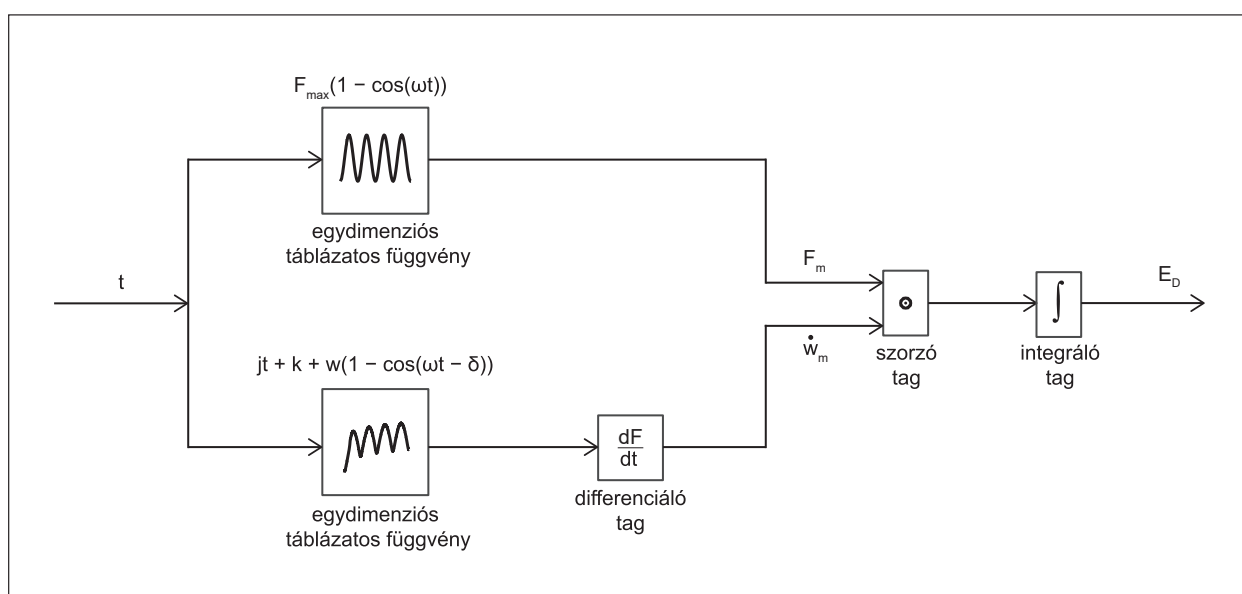
3.22. ábra Disszipált energia meghatározása Simulink környezetben
