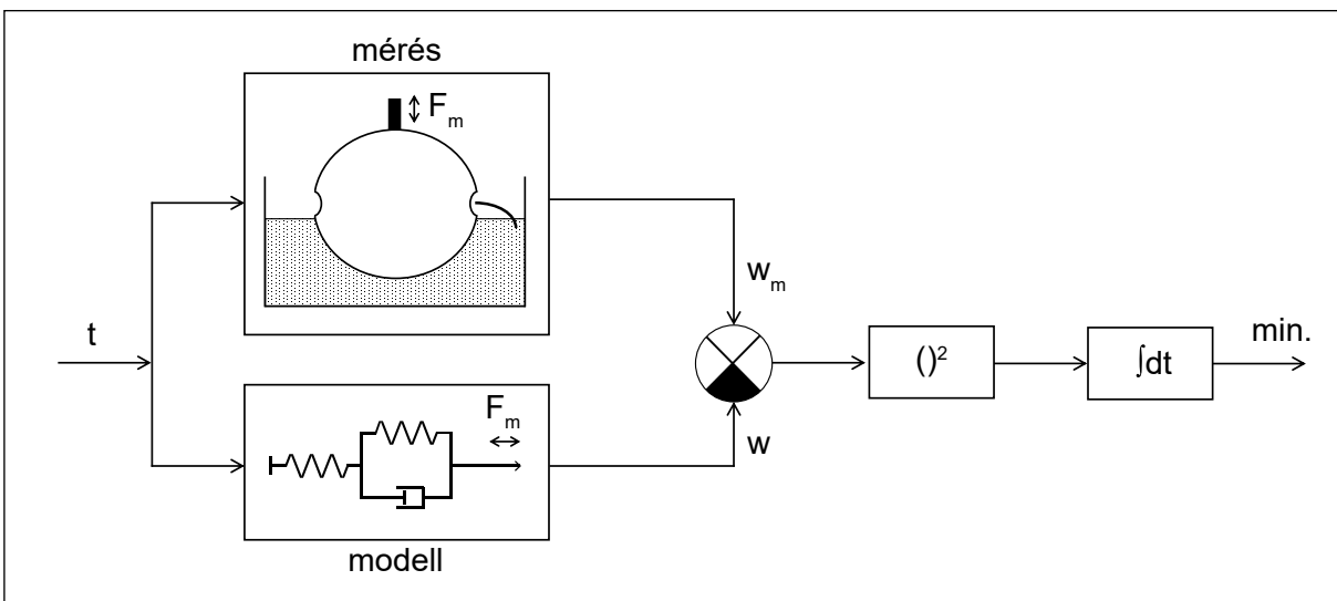
3.19. ábra A rendszerazonosítás hatásvázlata
