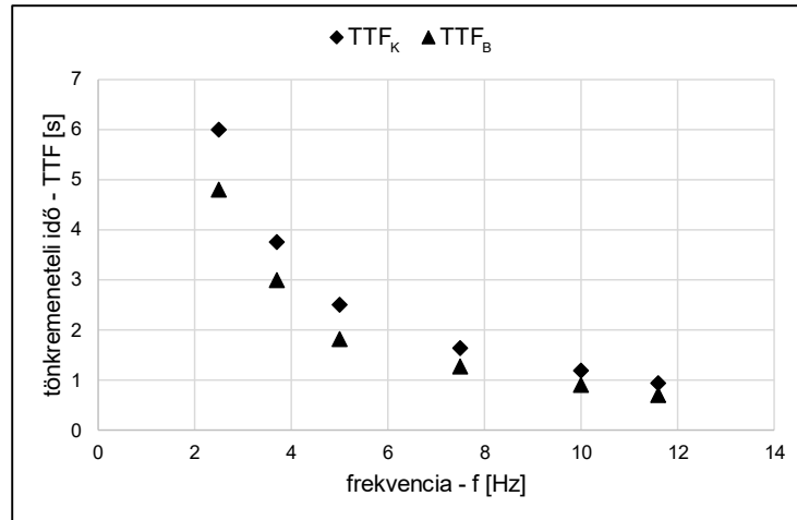
4.7. ábra Külső (TTF K ) és belső (TTF B ) tönkrementelig eltelt időtartamok frekvenciafüggése Golden Delicious almák esetén
