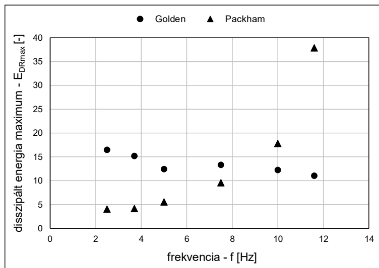
4.3. ábra A halmazódó disszipált energiák átlagértékeinek frekvenciafüggése
