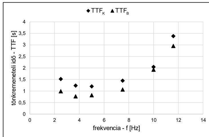
4.8. ábra Külső (TTF K ) és belső (TTF B ) tönkrementelig eltelt időtartamok frekvenciafüggése Packham körték esetén
